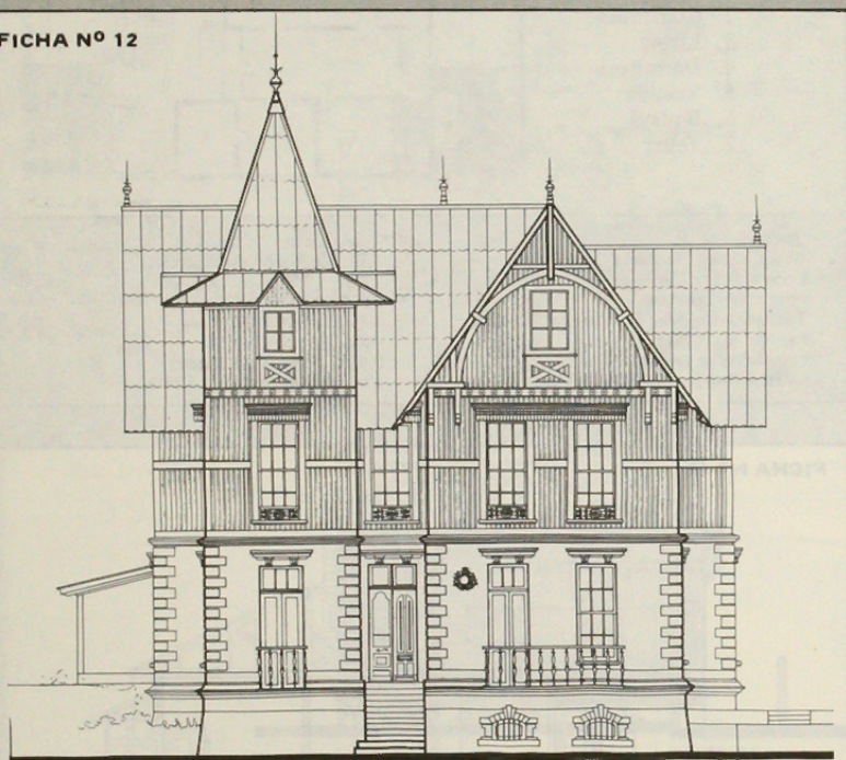
ELEVACION PRINCIPAL
