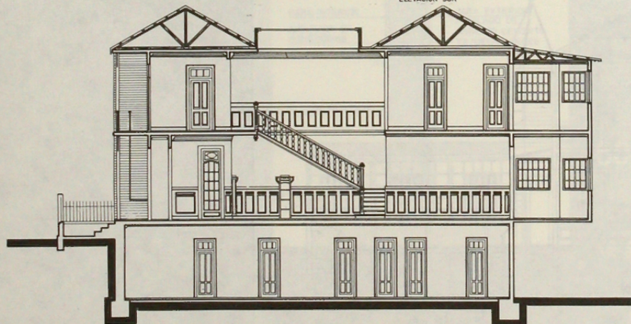
CORTE LONGITUDINAL
