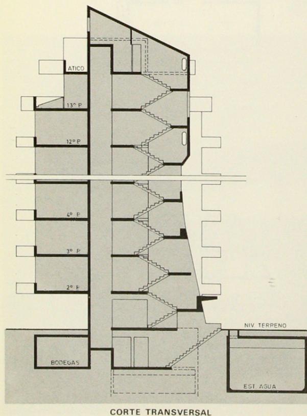
CORTE TRANSVERSAL
