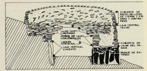
PERFIL TRANSVERSAL
