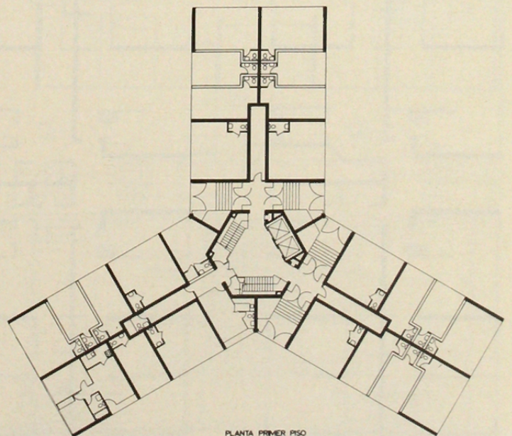
PLANTA PRIMER PISO
