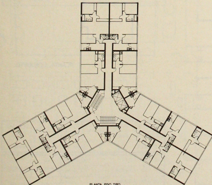
PLANTA PISO TIPO
