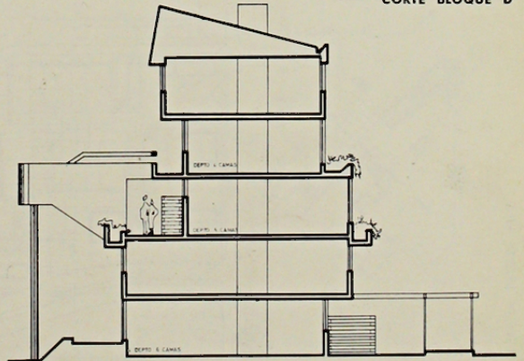
CORTE BLOQUE B
