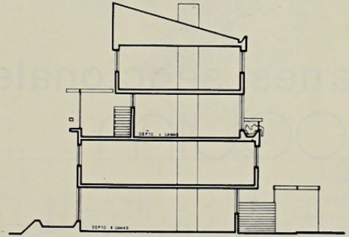
CORTE BLOQUE D
