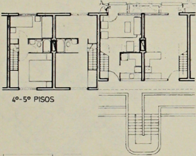
PLANTAS DEPARTAMENTOS BLOQUE TIPO D
